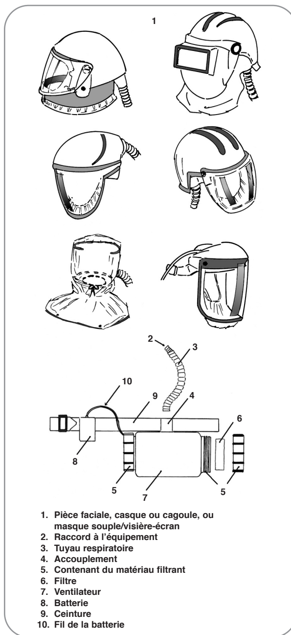
Figure 7 – Appareils de protection respiratoire motorisés avec pièce faciale non hermétique
